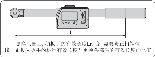
扭矩修正
